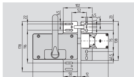
Actuator AZ 16-ST330
